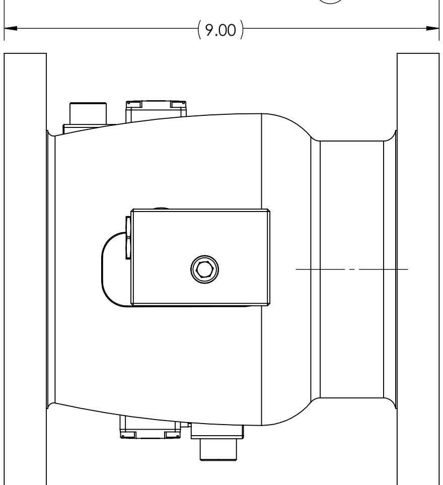
P/N PCV290FF SHOWN
