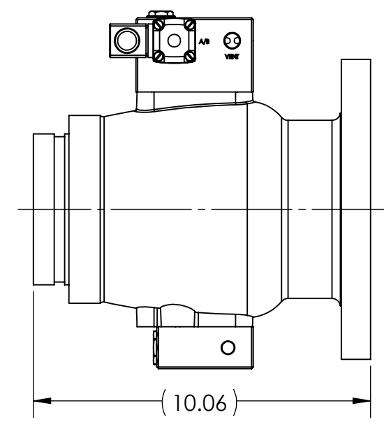
P/N PCV290VF SHOWN
