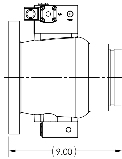
P/N PCV290FV SHOWN
