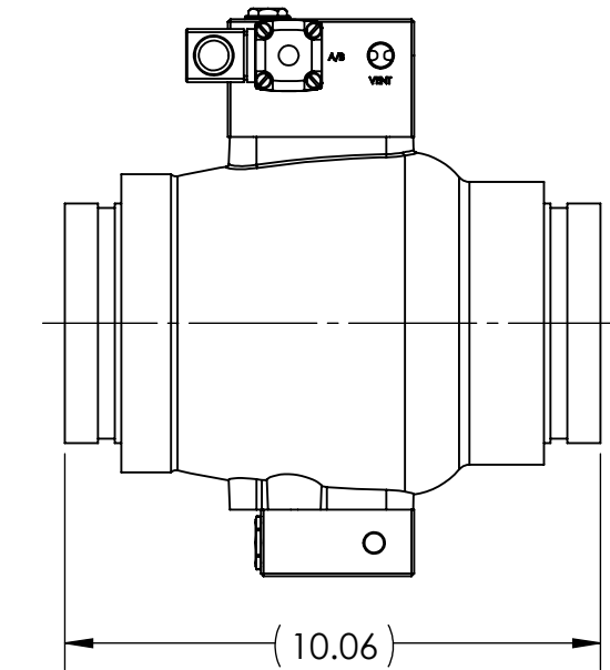
P/N PCV290VV SHOWN
